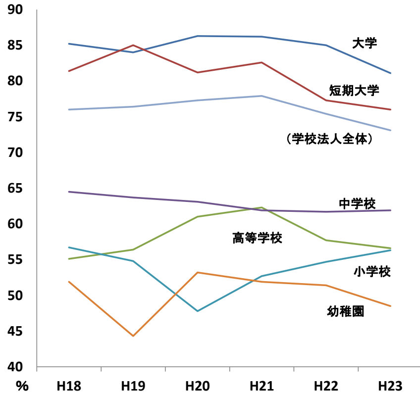
① 学生生徒等納付金比率 \frac{\text{学生生徒等納付金}}{\text{帰属収入}}
